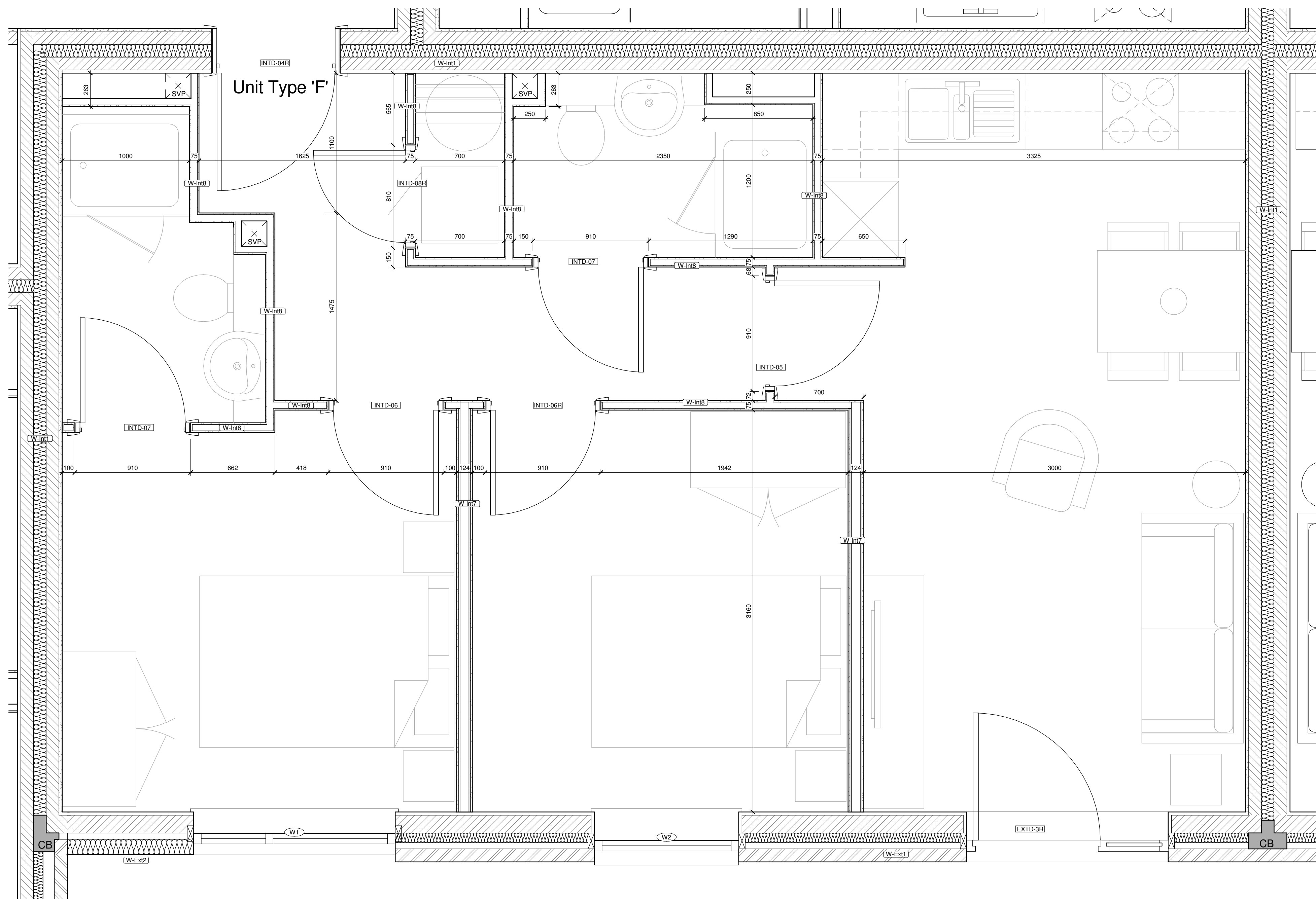
1 Unit Type 'F' 1 : 20
